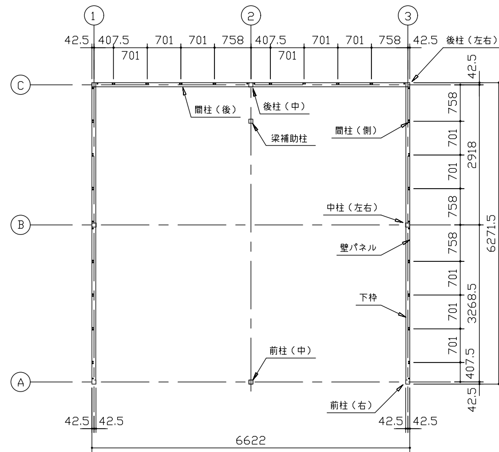
平面図 (S=1/80)
