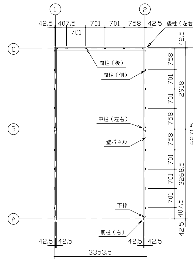
平面図 (S=1/80)
