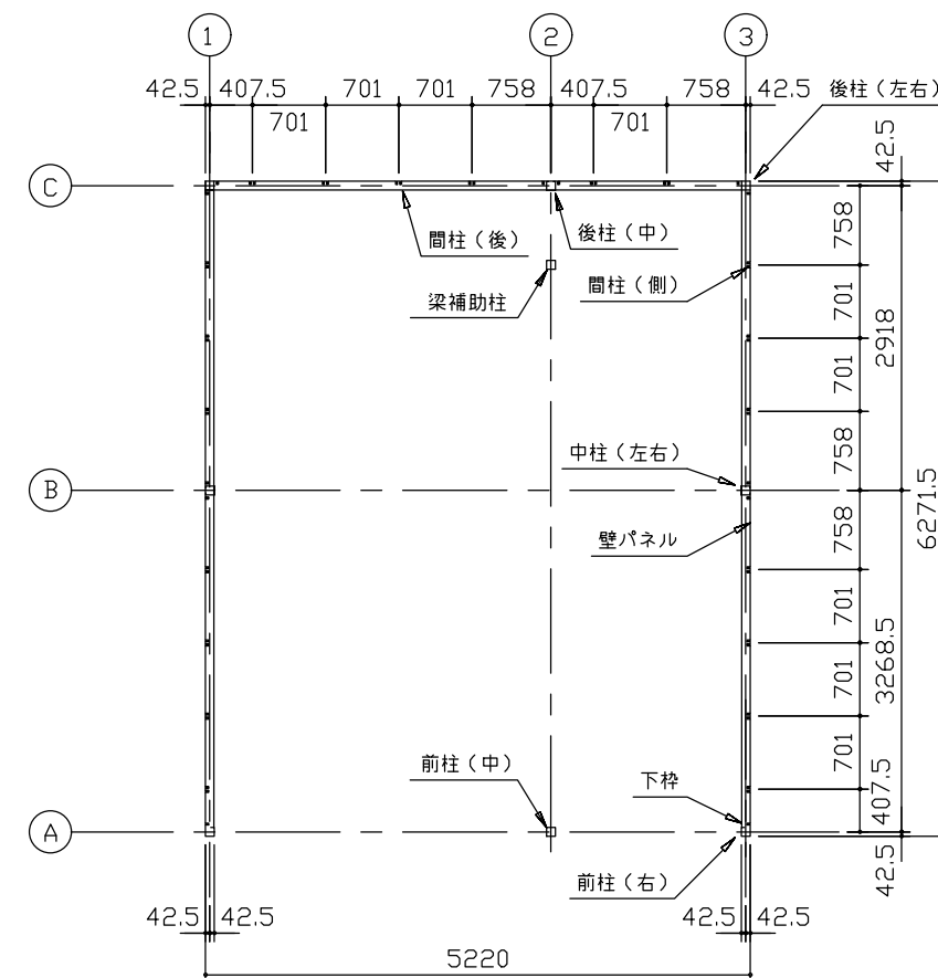
平面図 (S=1/80)
