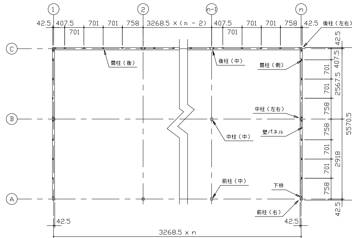
平面図 (S=1/80)
