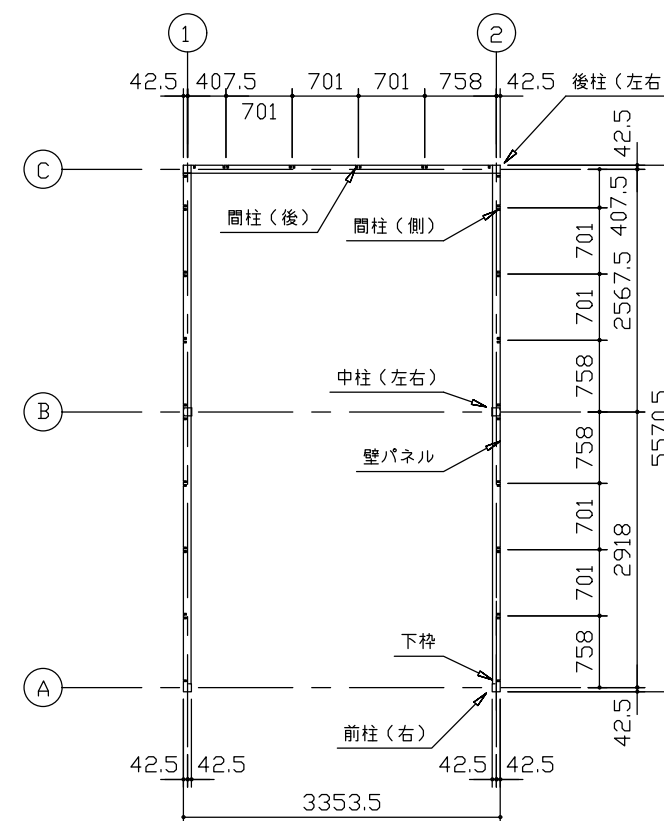
平面図 (S=1/80)
