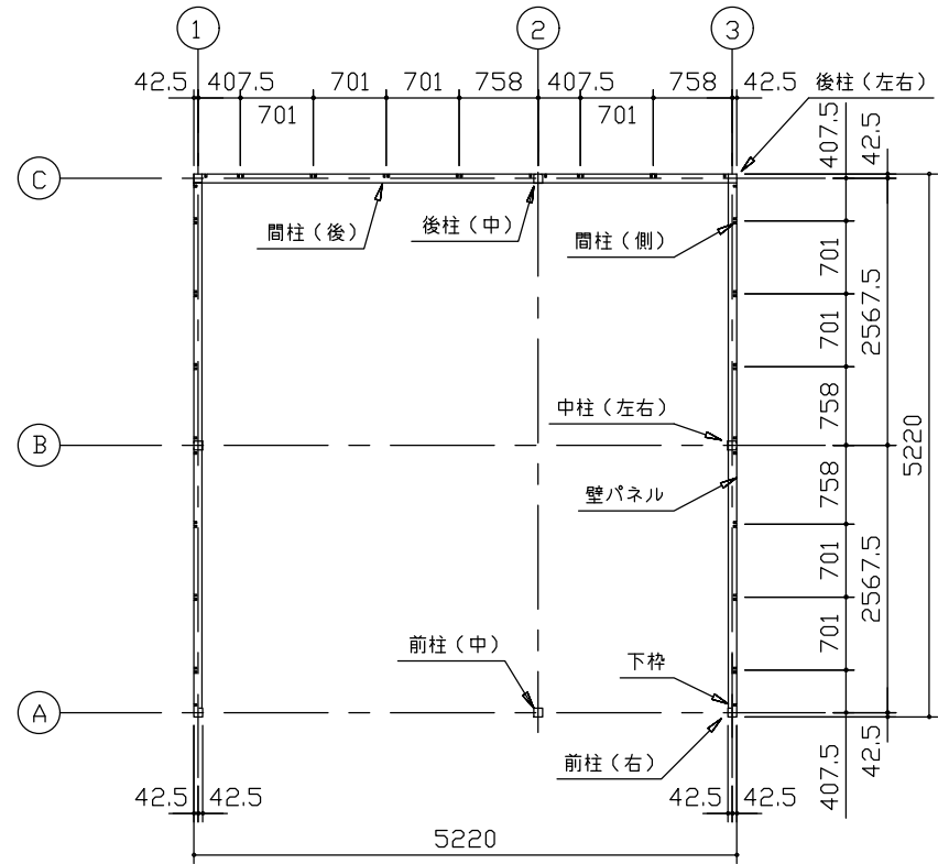
平面図 (S=1/80)
