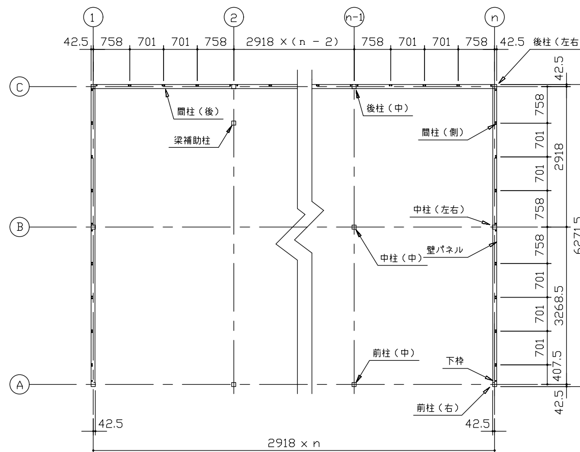
平面図 (S=1/80)
