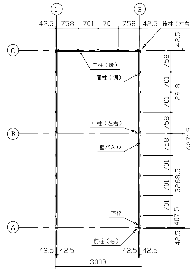
平面図 (S=1/80)
