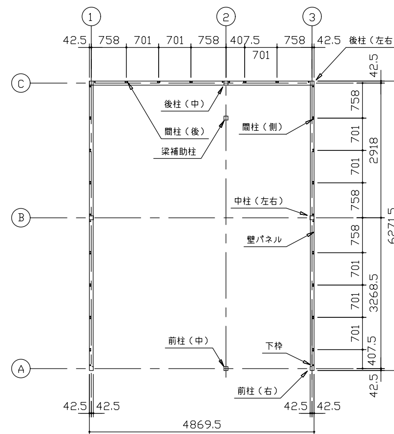
平面図 (S=1/80)
