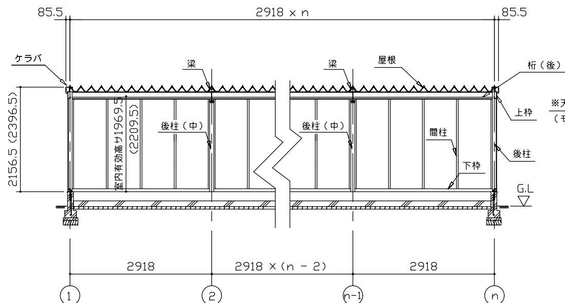
正 面 断 面 图 ( S=1/80 )
