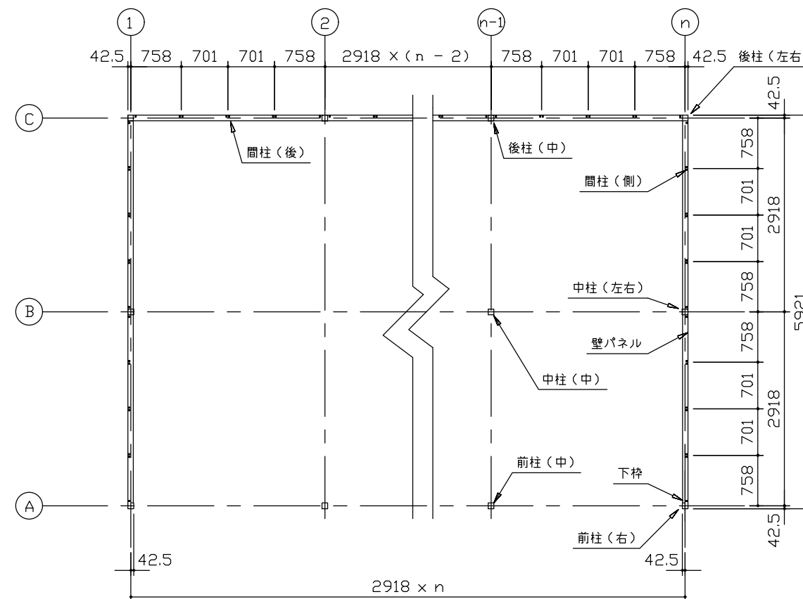
平面図 (S=1/80)
