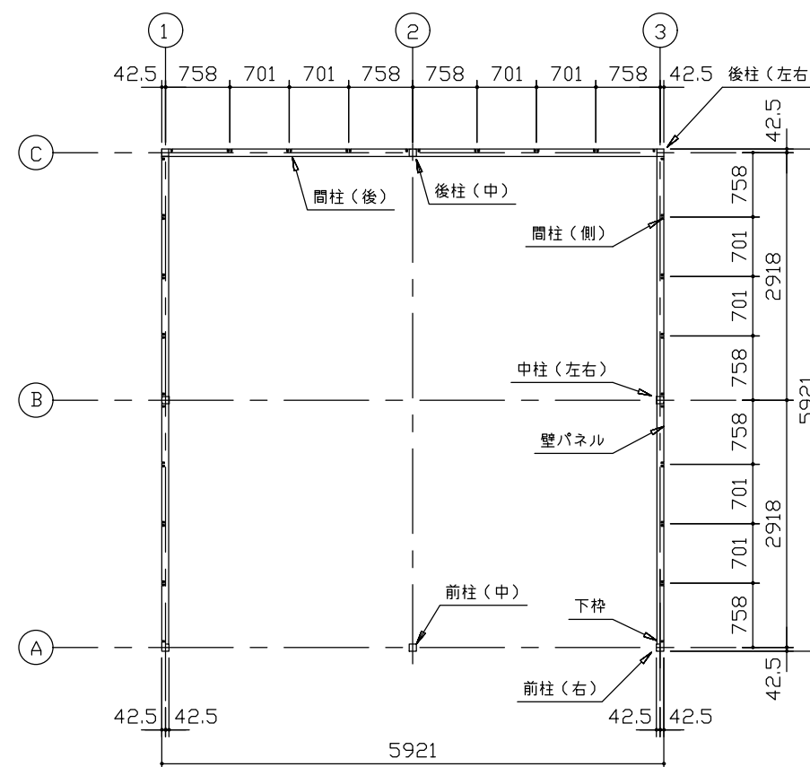
平面図 (S=1/80)
