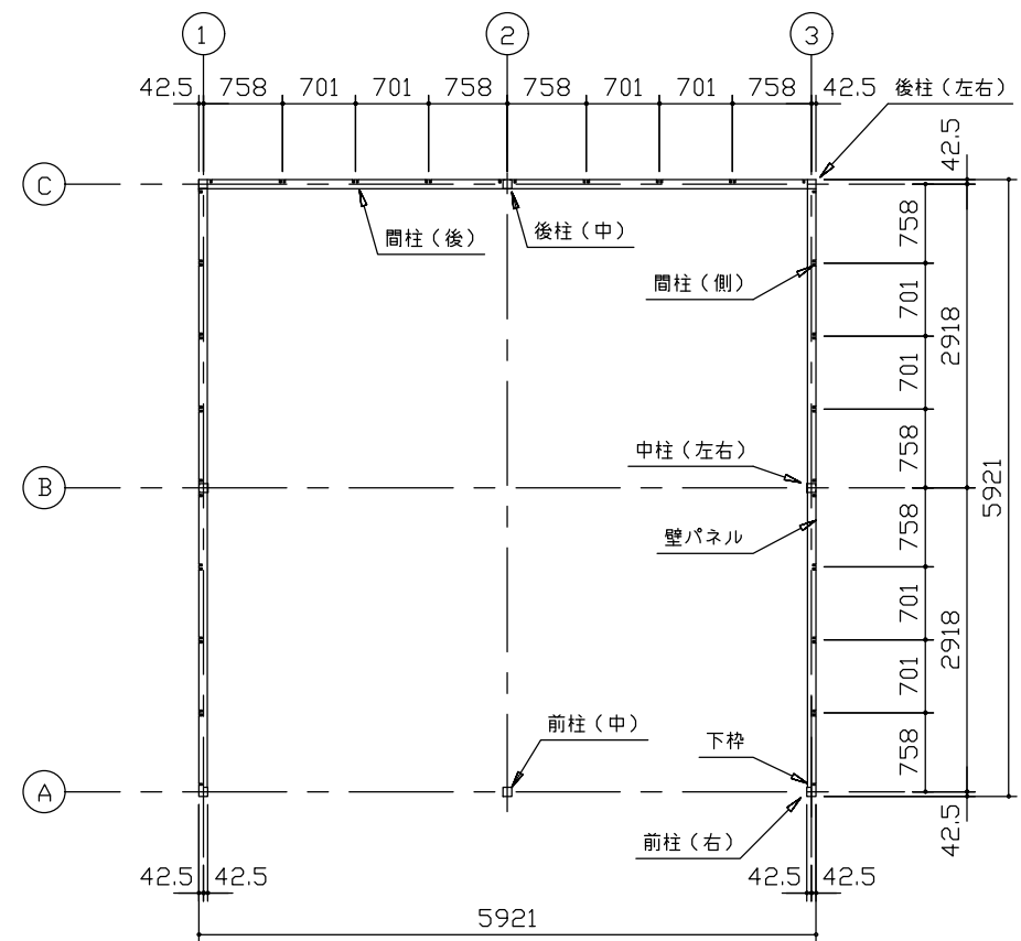
平面図 (S=1/80)
