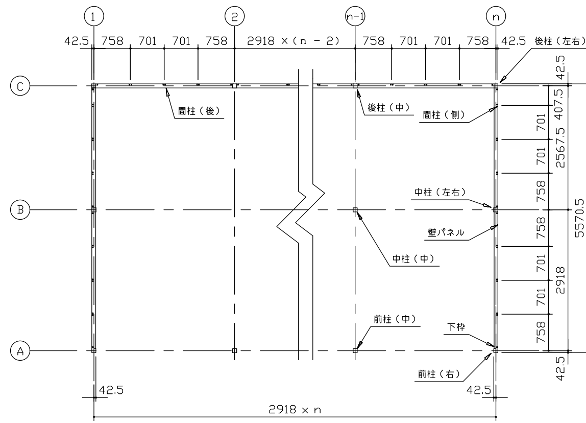
平面図 (S=1/80)
