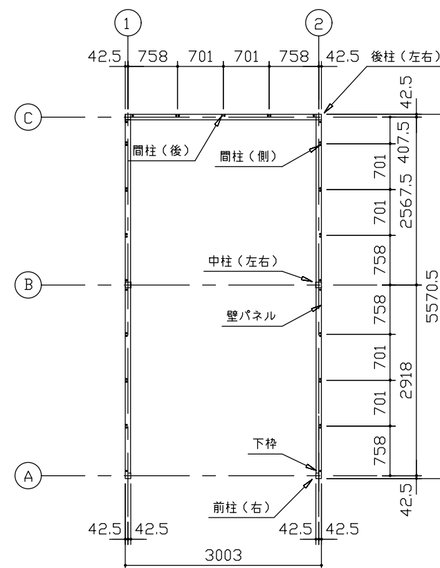
平面図 (S=1/80)
