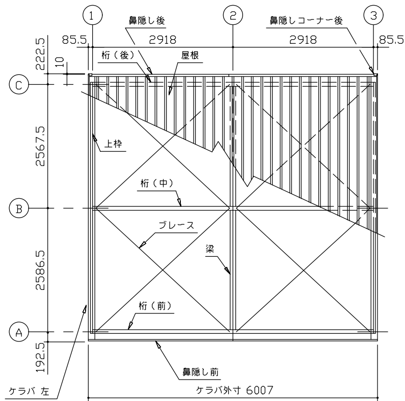
小屋伏図 (S=1/80)
