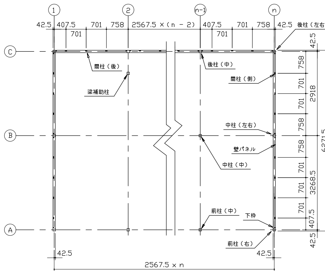
平面図 (S=1/80)
