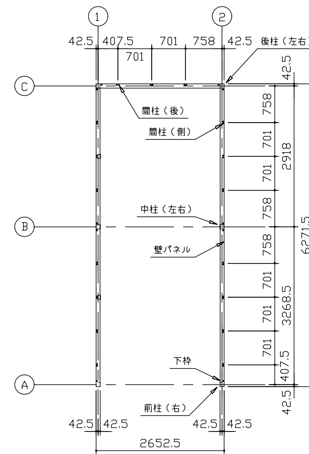
平面図 (S=1/80)
