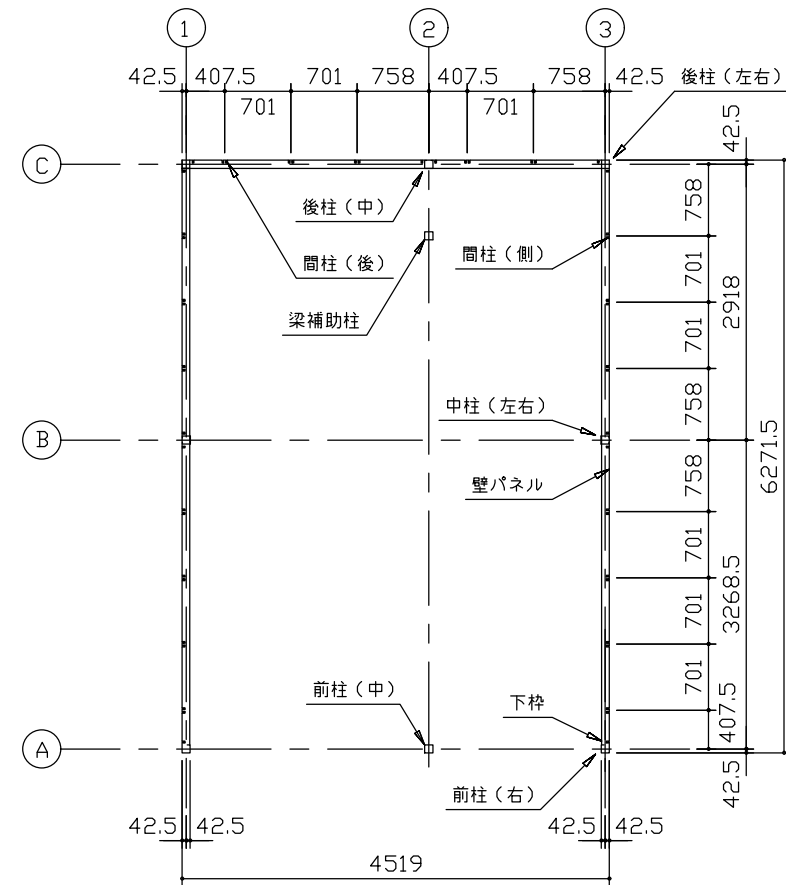
平面図 (S=1/80)
