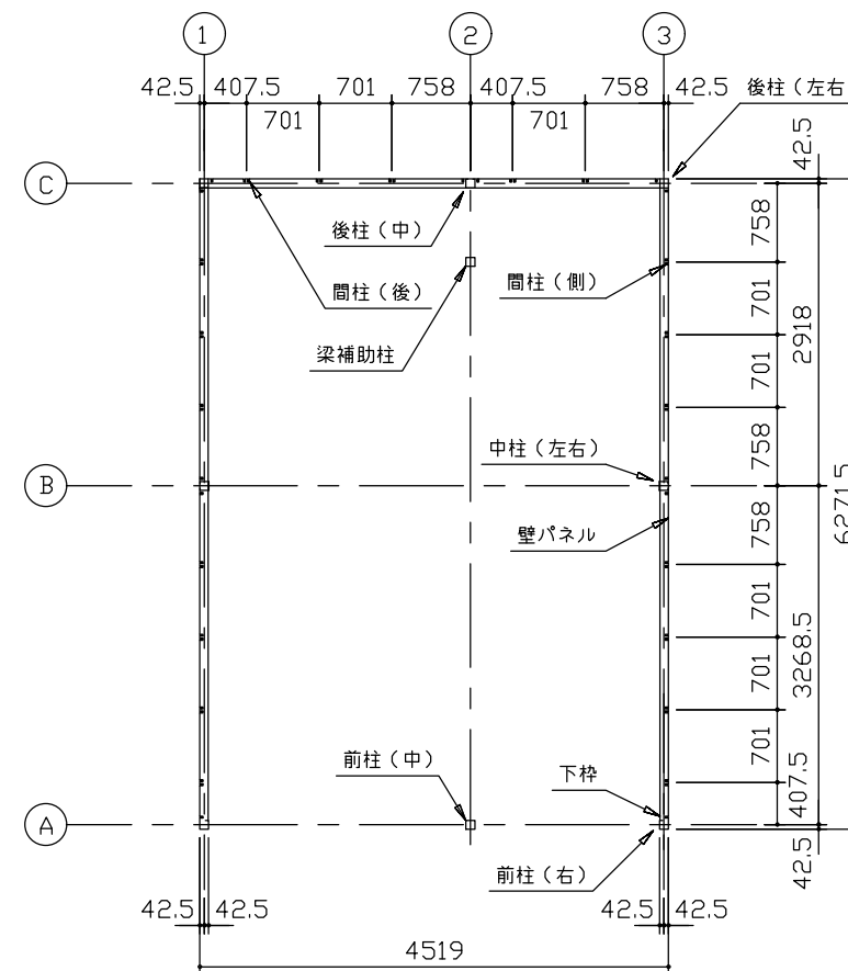
平面図 (S=1/80)
