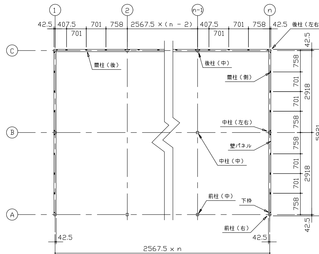
平面図 (S=1/80)
