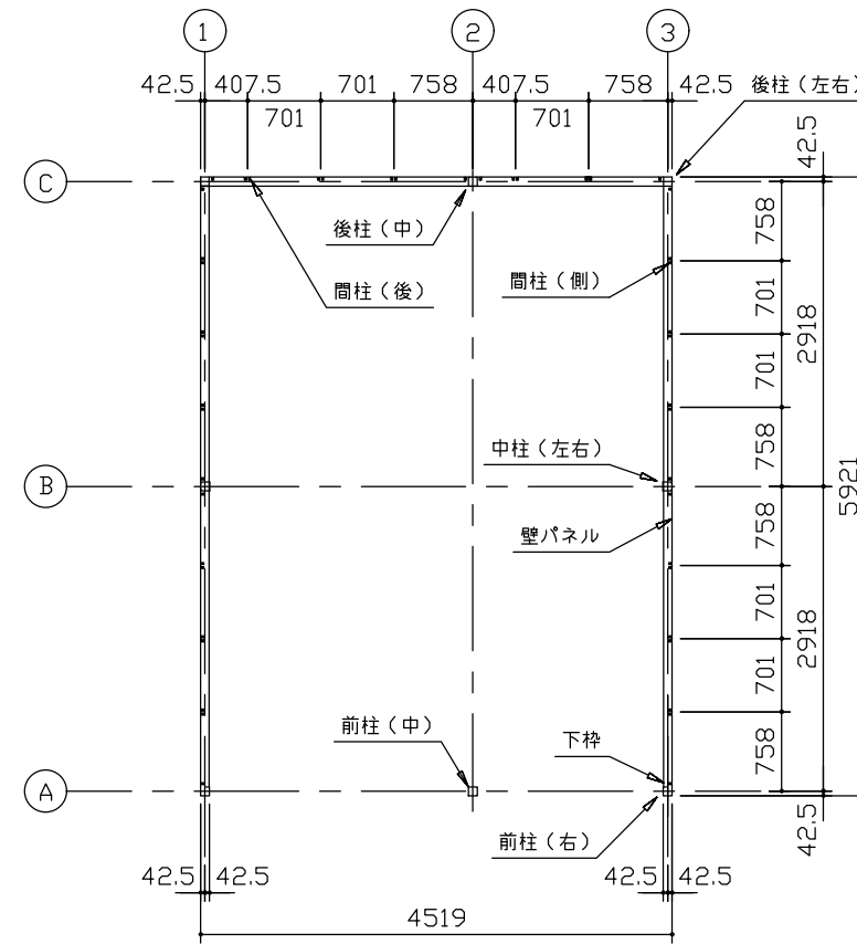
平面図 (S=1/80)
