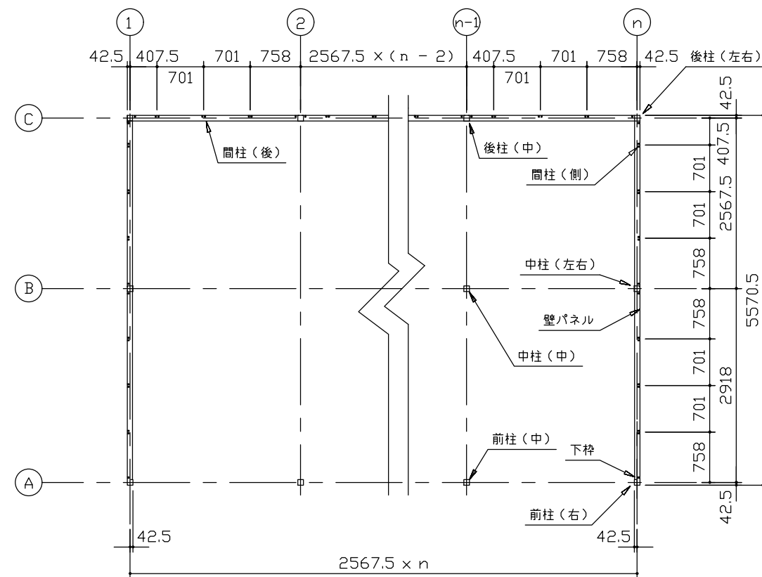
平面図 (S=1/80)
