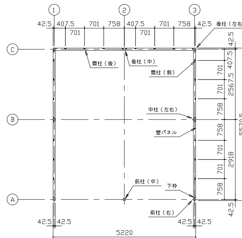
平面図 (S=1/80)
