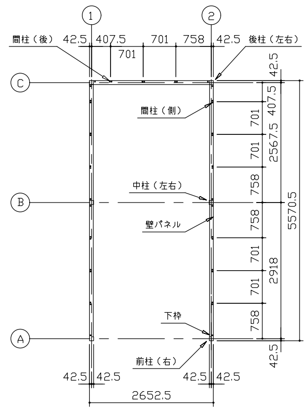
平面図 (S=1/80)
