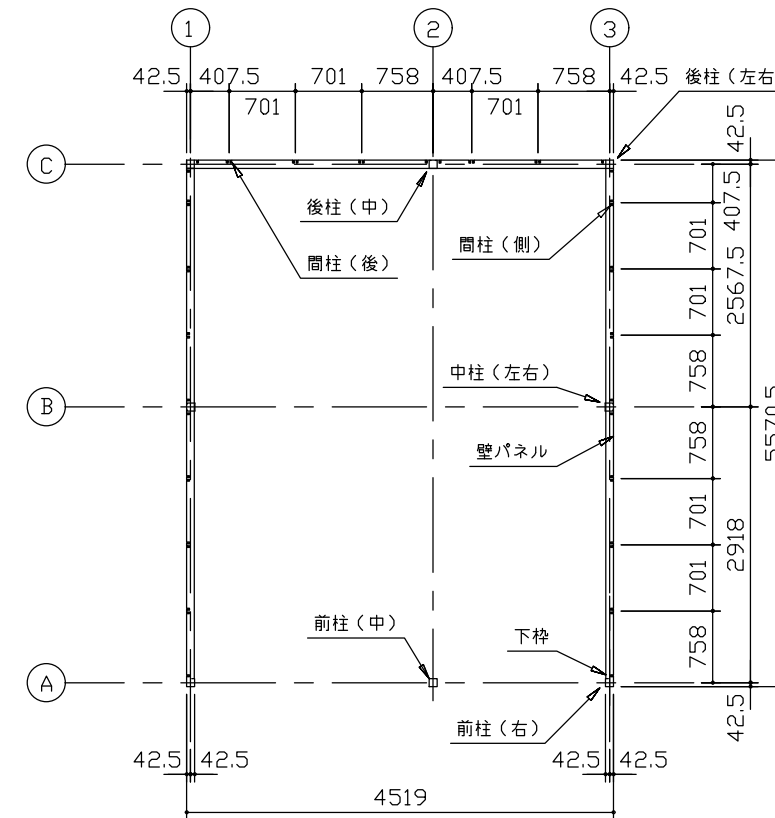
平面図 (S=1/80)
