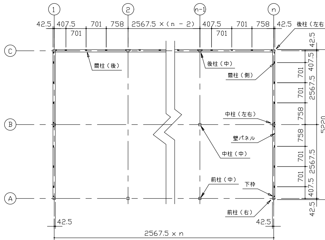
平面図 (S=1/80)
