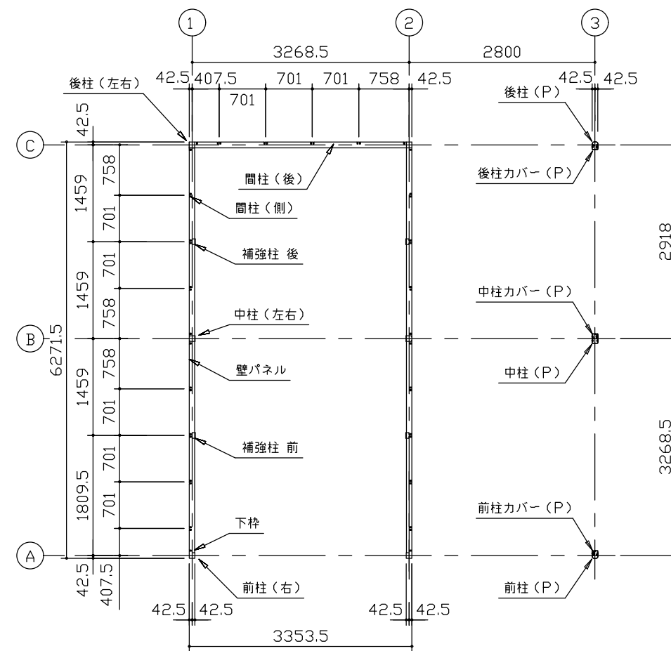
平面図 (S=1/80)
