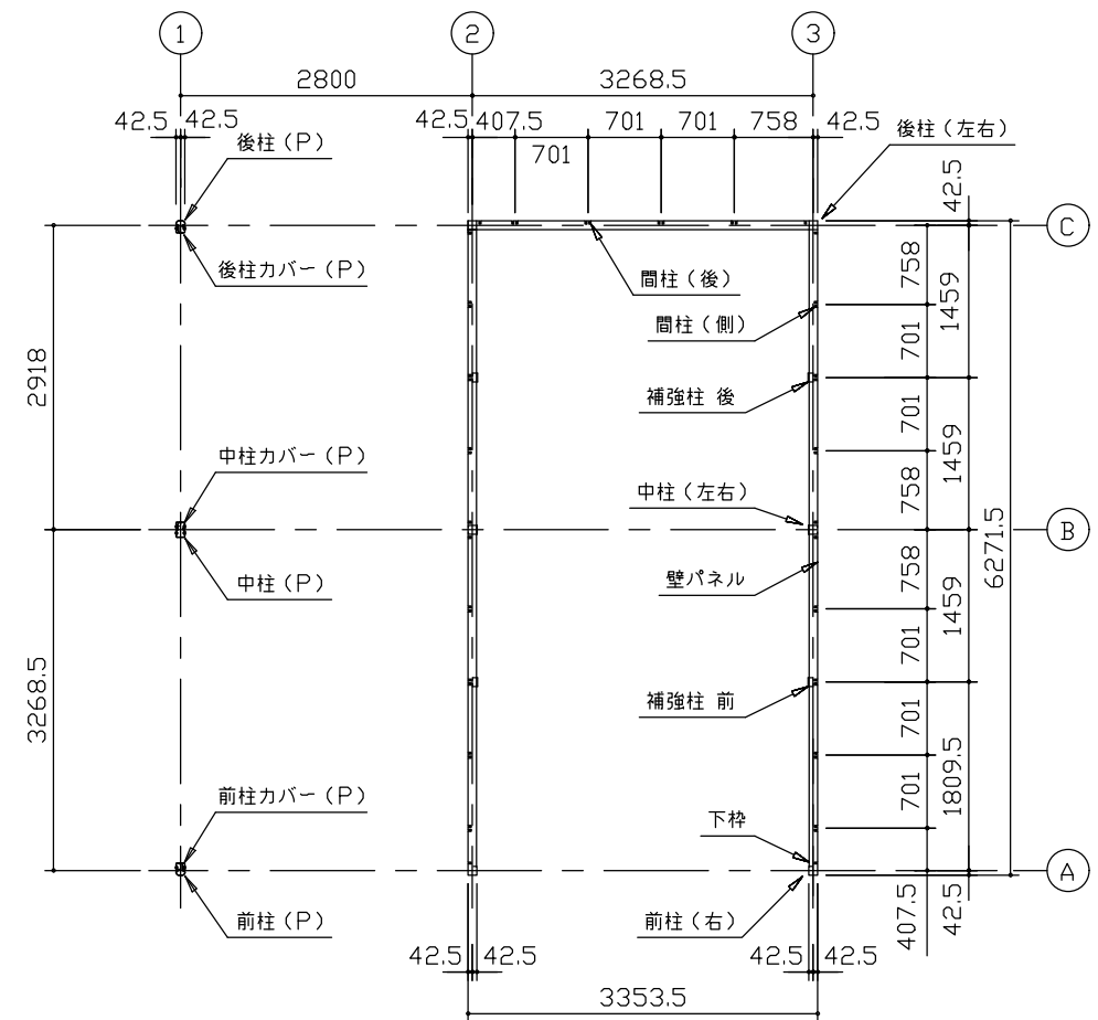
平面図 (S=1/80)
