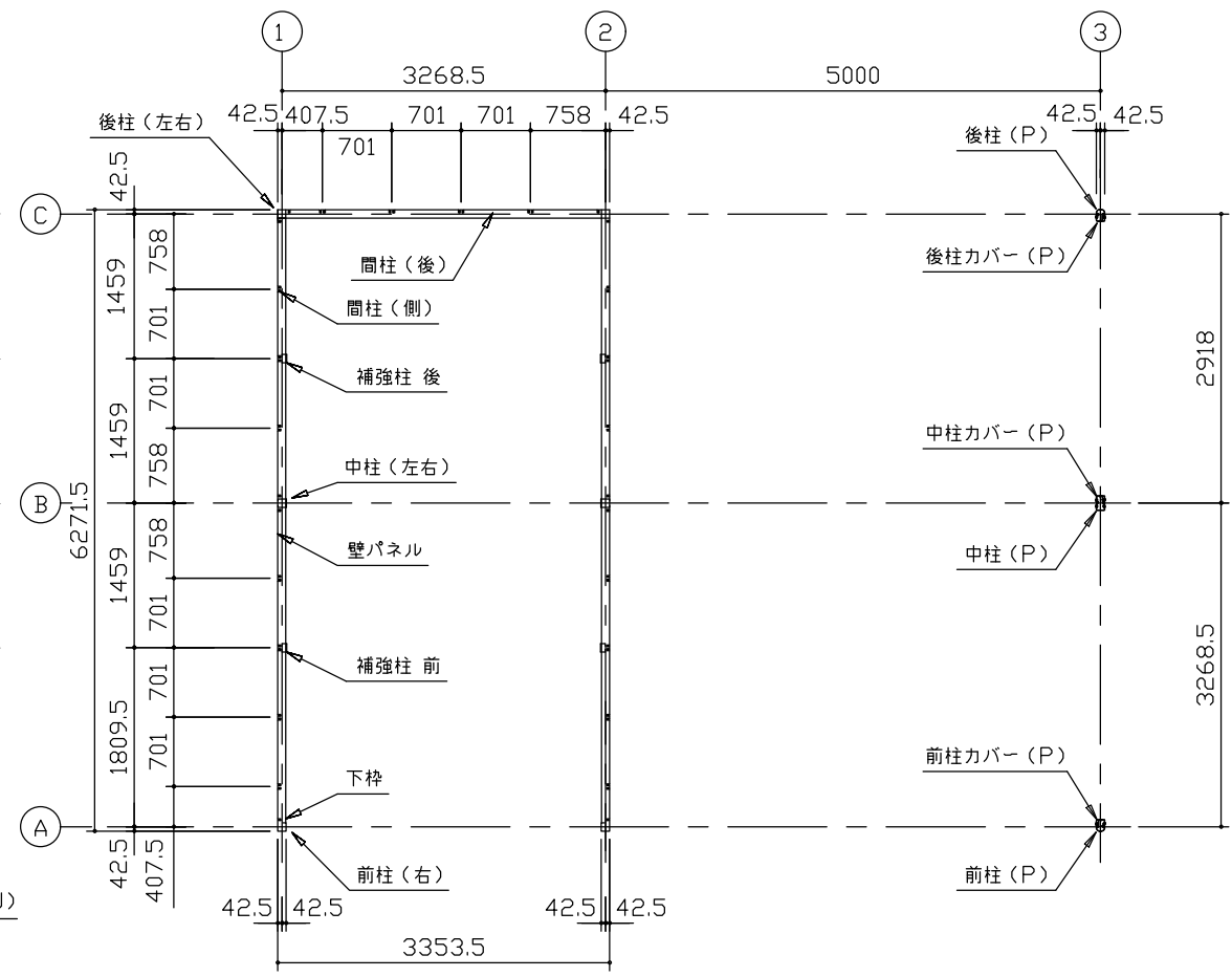
平面図 (S=1/80)
