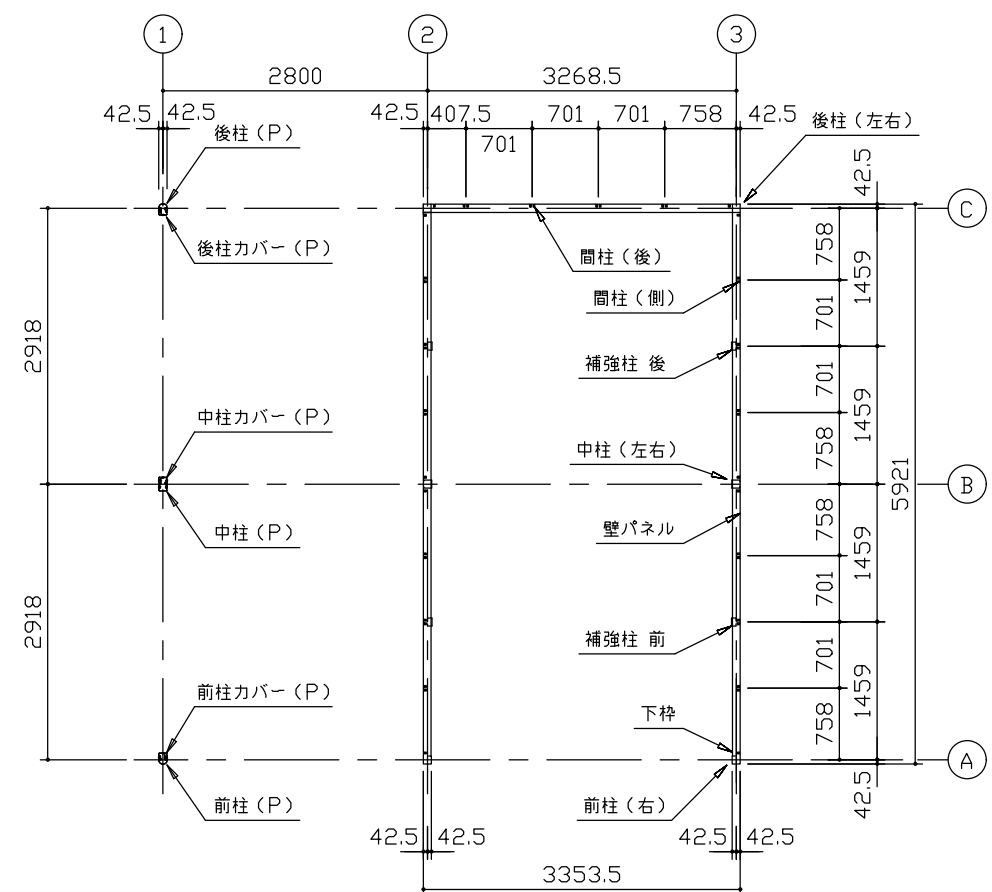
平面図 (S=1/80)
