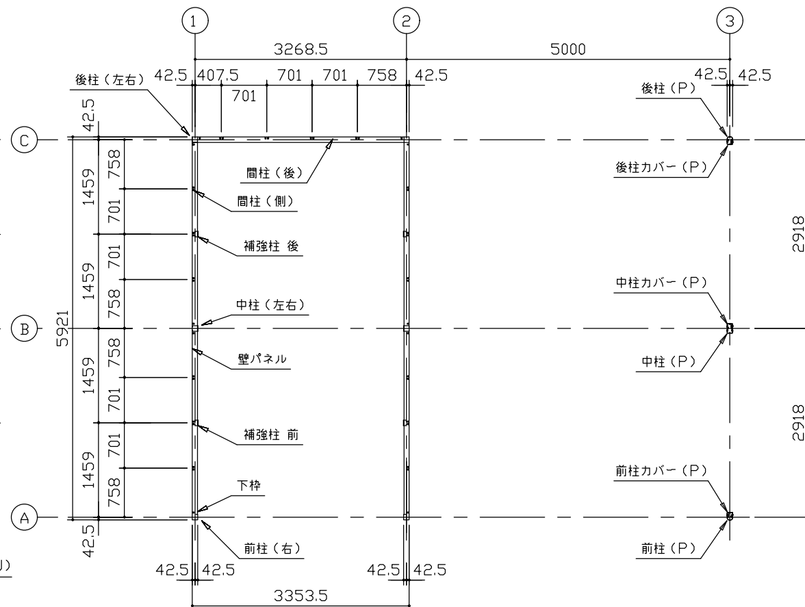
平面図 (S=1/80)
