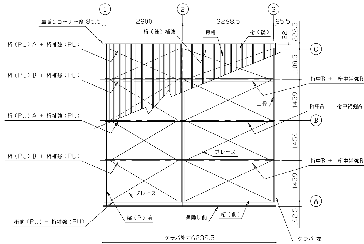
小屋伏図 (S=1/80)
