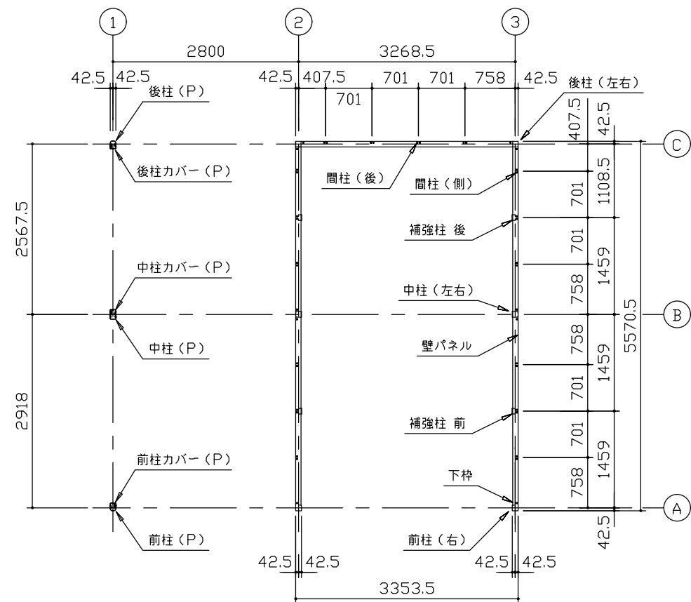
平面図 (S=1/80)
