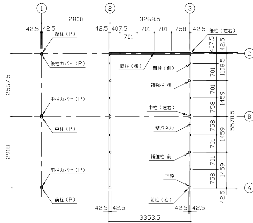
平面図 (S=1/80)
