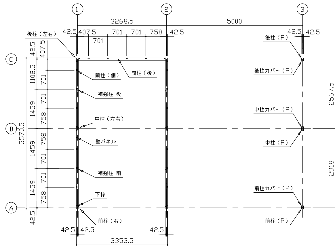
平面図 (S=1/80)
