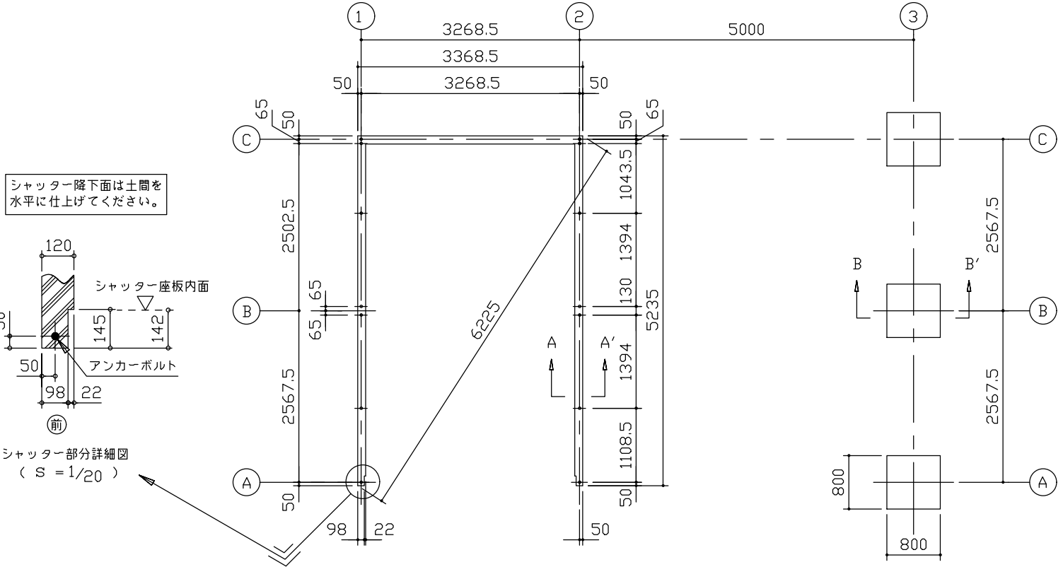
布基礎伏図 (S=1/80)
