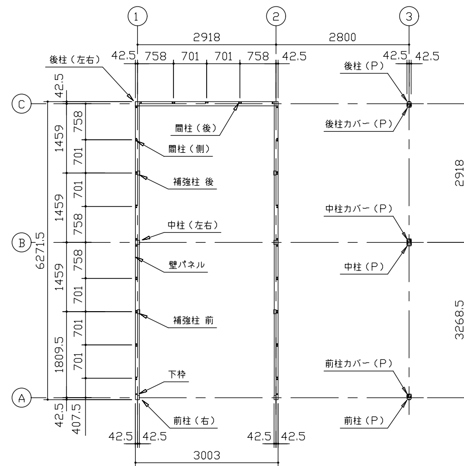
平面図 (S=1/80)
