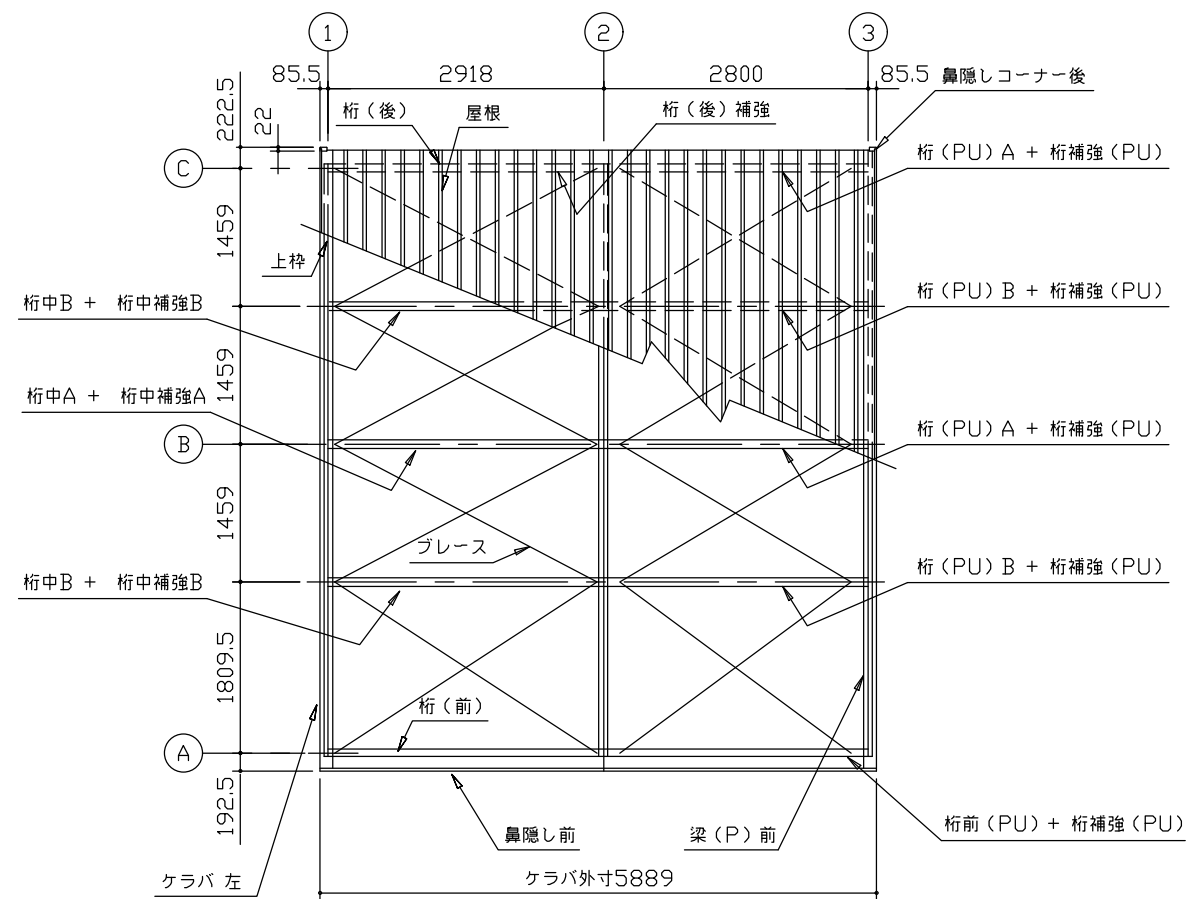
小屋伏図 (S=1/80)
