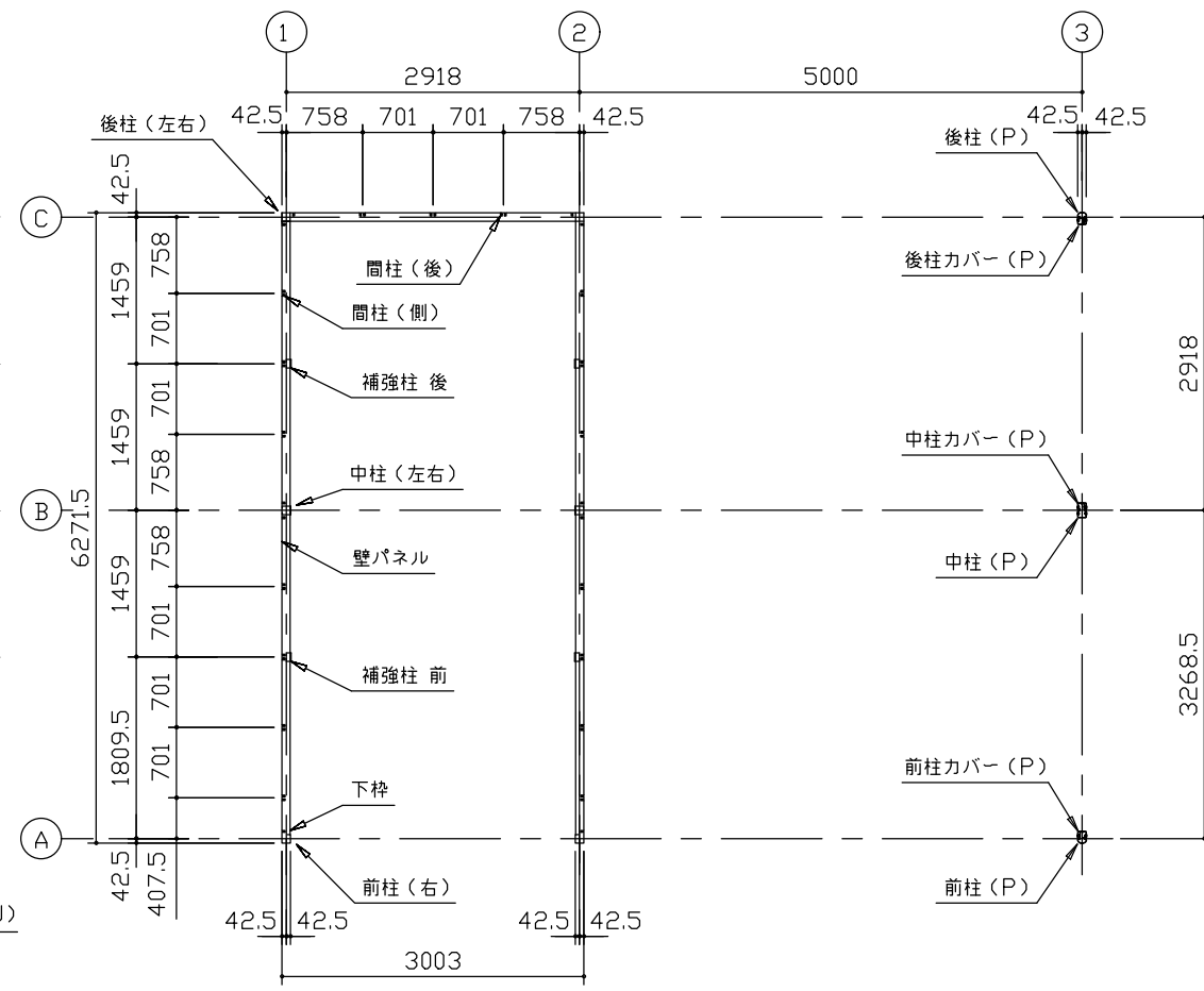
平面図 (S=1/80)
