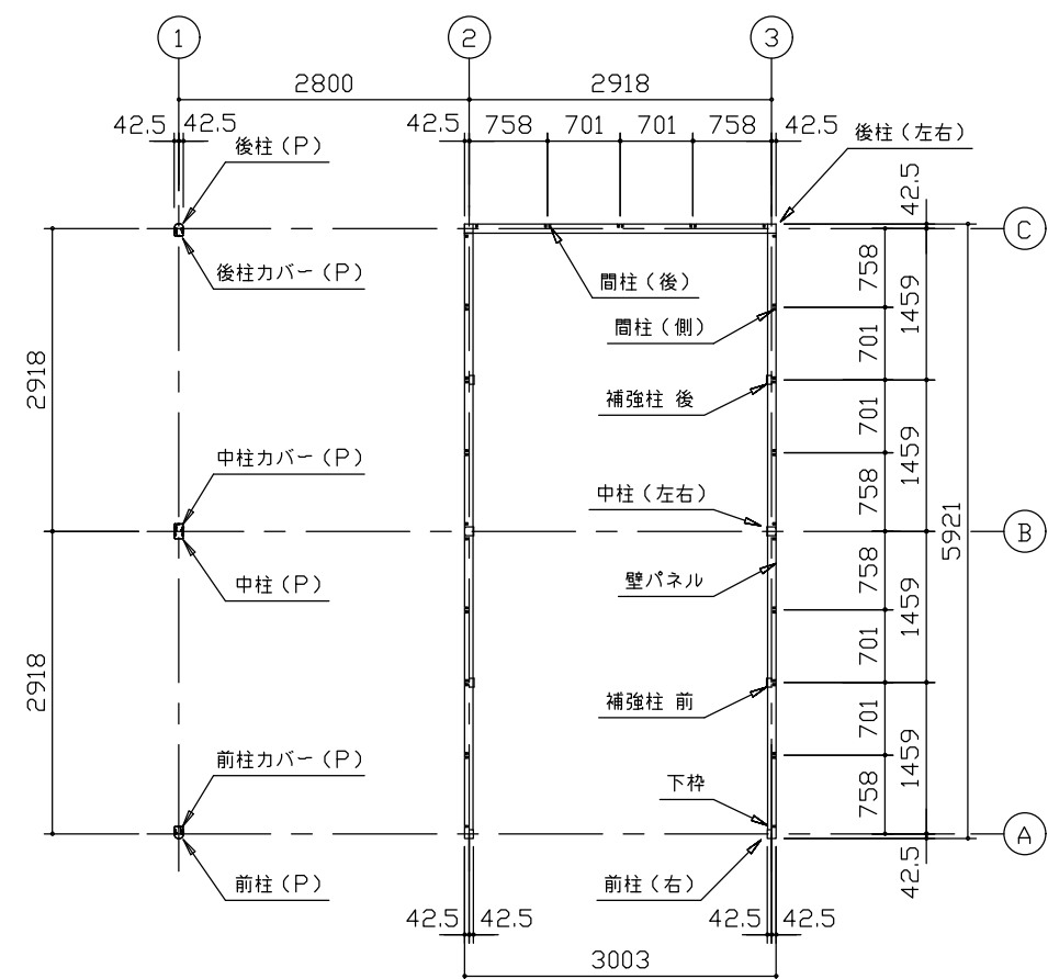
平面図 (S=1/80)
