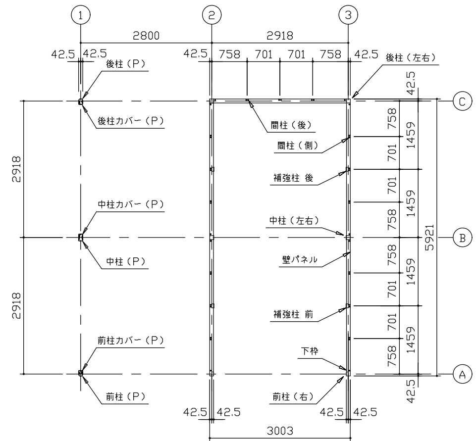
平面図 (S=1/80)
