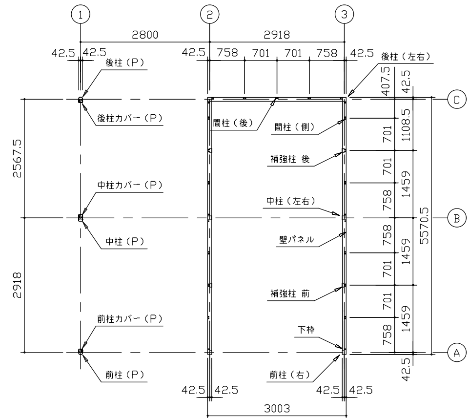
平面図 (S=1/80)
