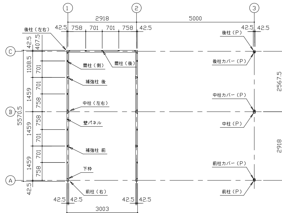
平面図 (S=1/80)
