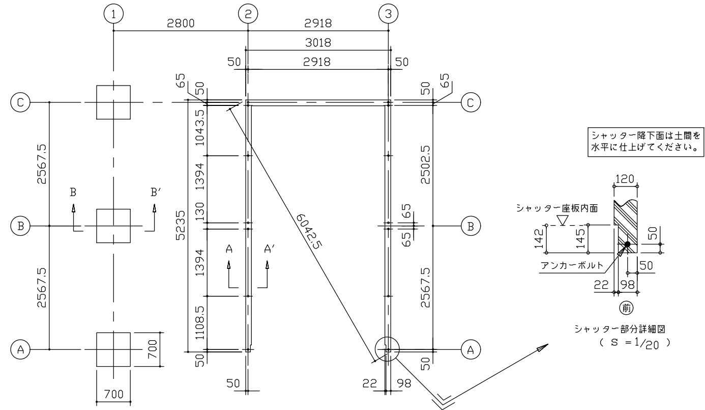
布基礎伏図 (S=1/80)
