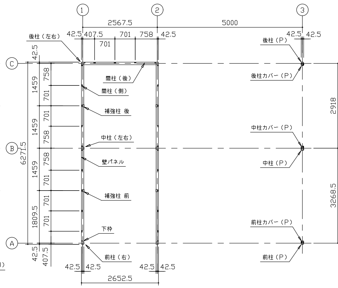
平面図 (S=1/80)
