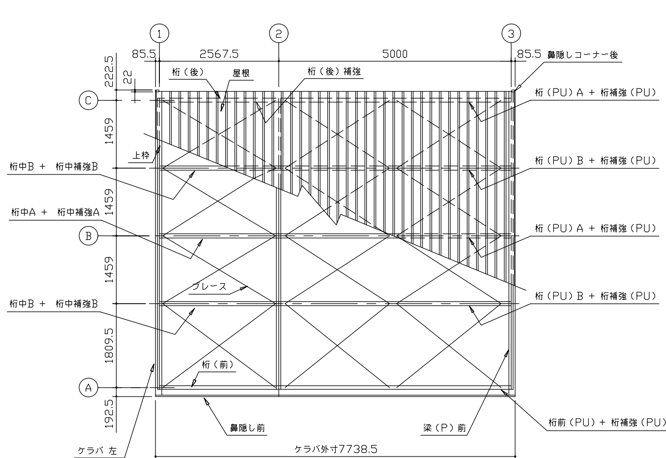
小屋伏図 (S=1/80)
