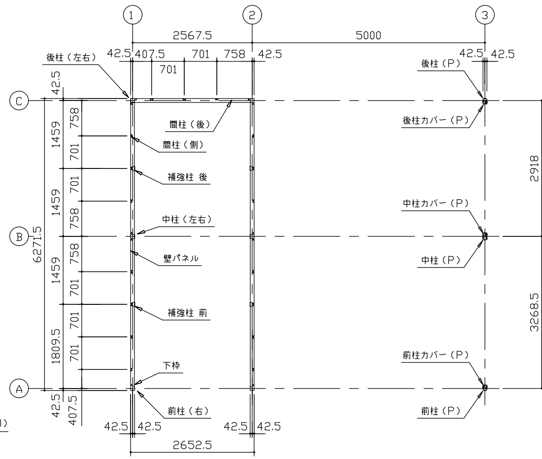
平面図 (S=1/80)
