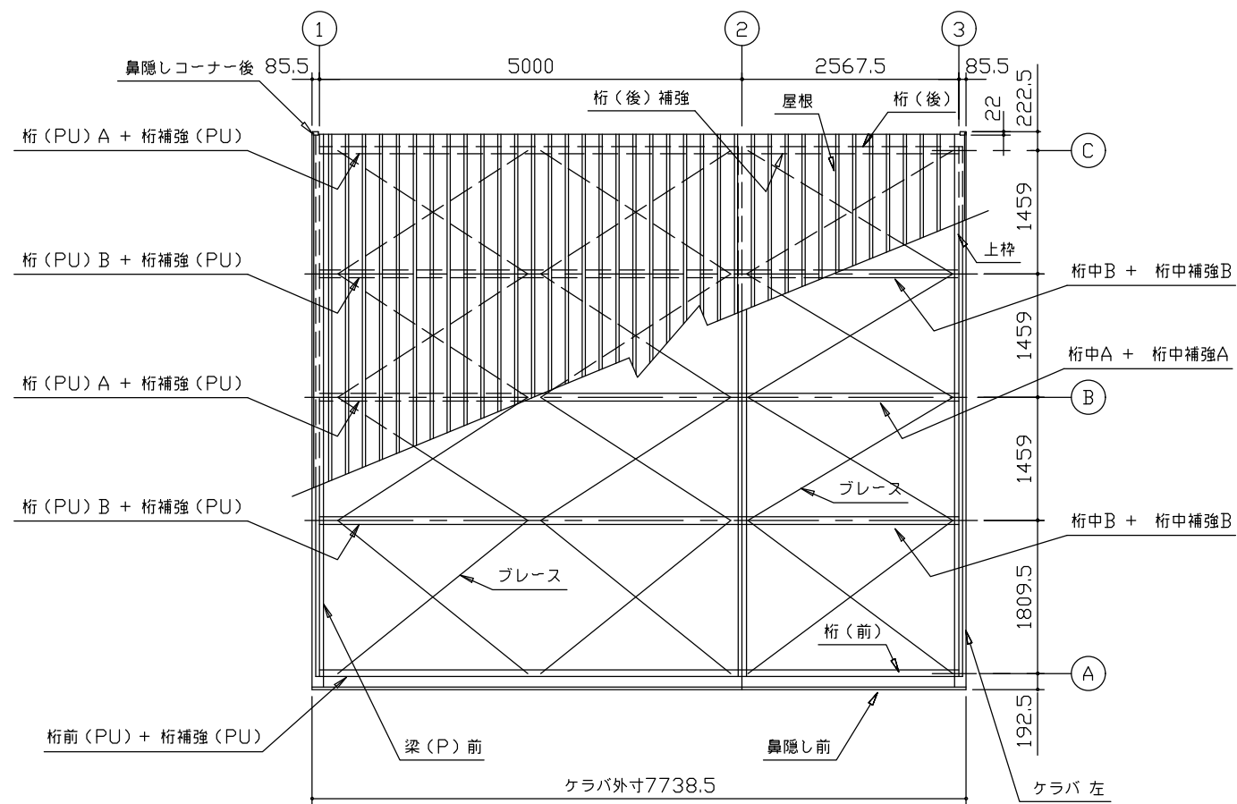
小屋伏図 (S=1/80)
