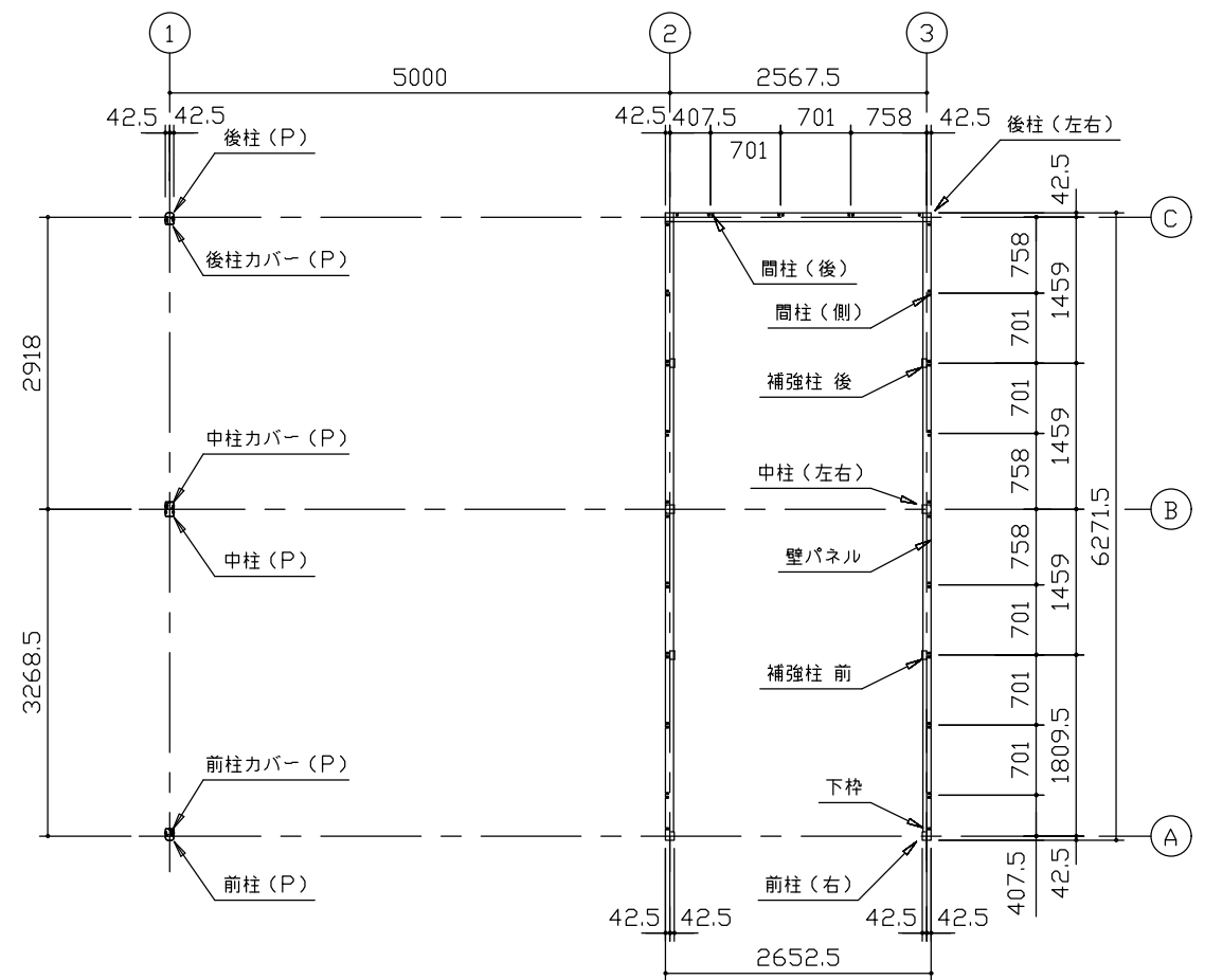
平面図 (S=1/80)
