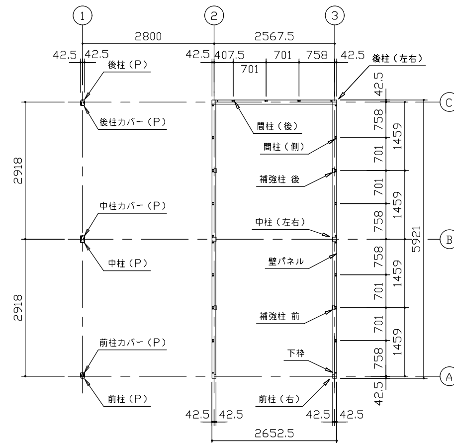
平面図 (S=1/80)
