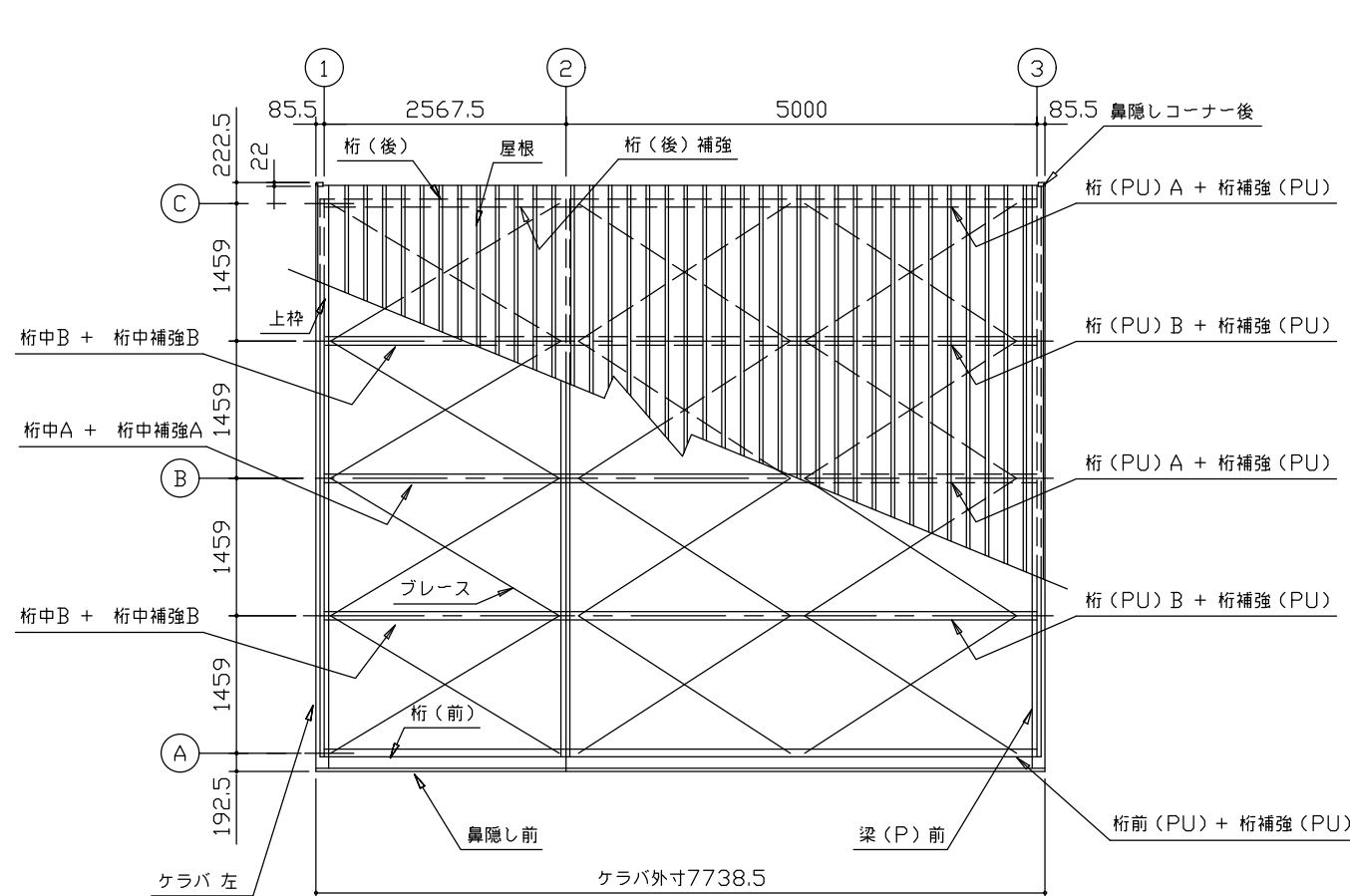
小屋伏図 (S=1/80)
