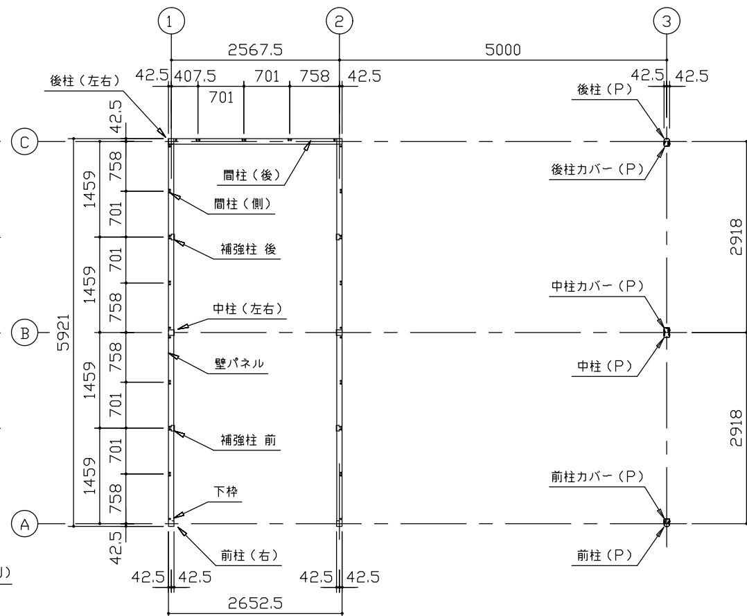
平面図 (S=1/80)
