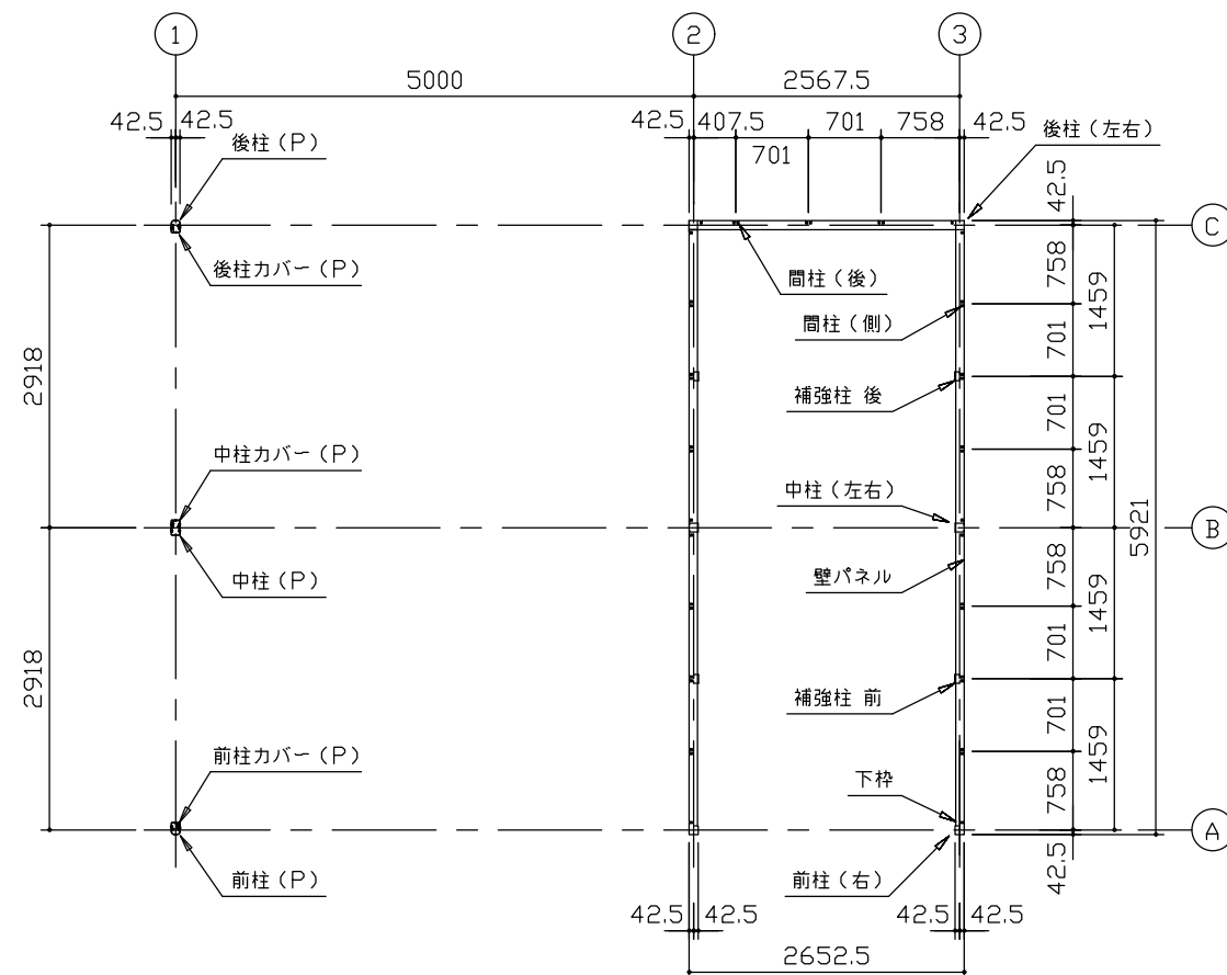
平面図 (S=1/80)
