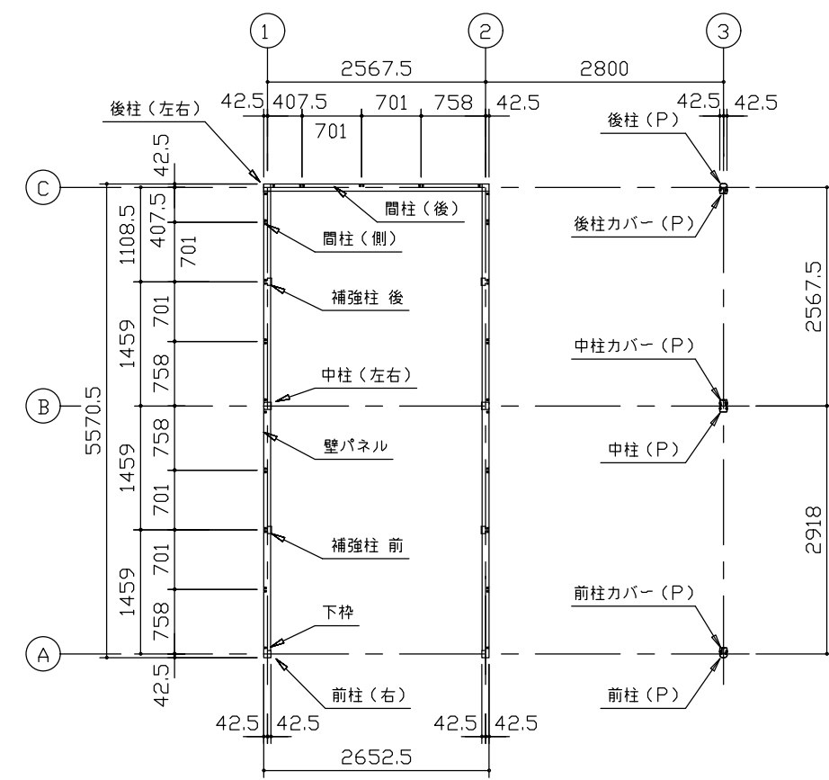
平面図 (S=1/80)
